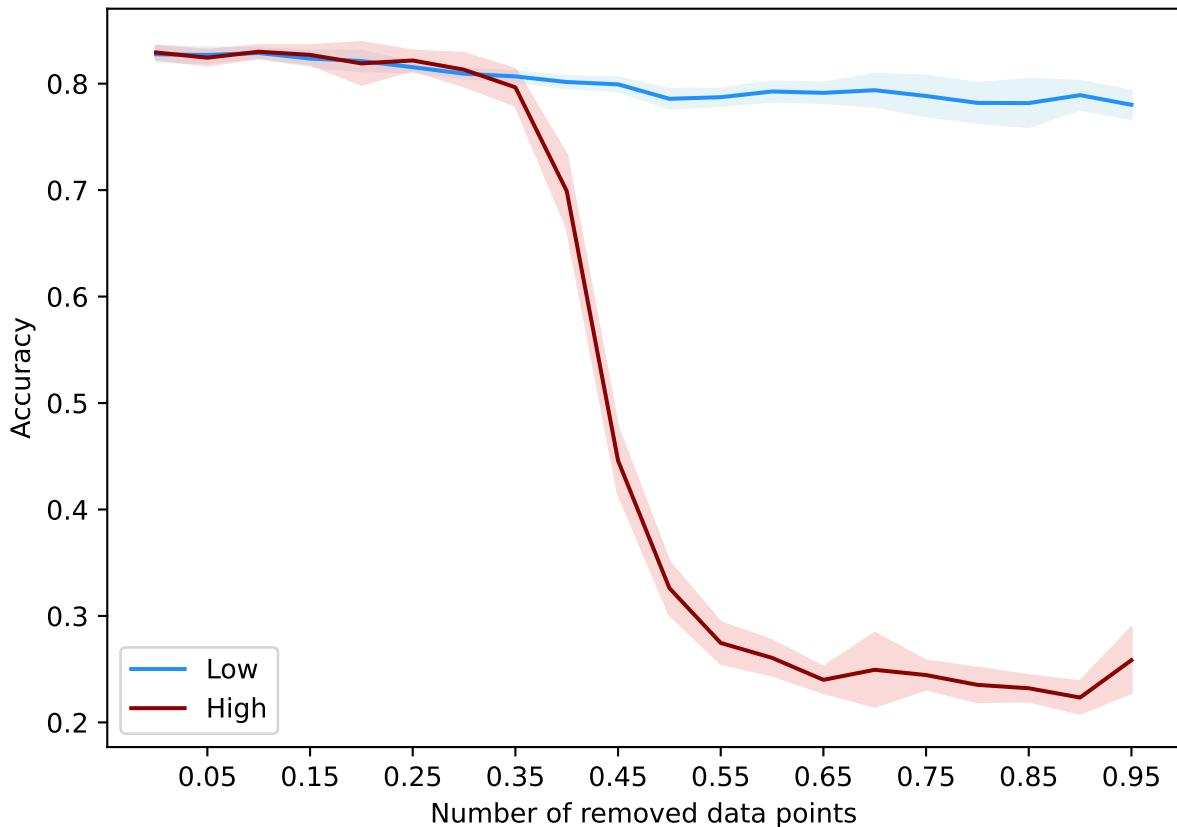
DataOob(1000, epochs=15) - imdb-embeddings
